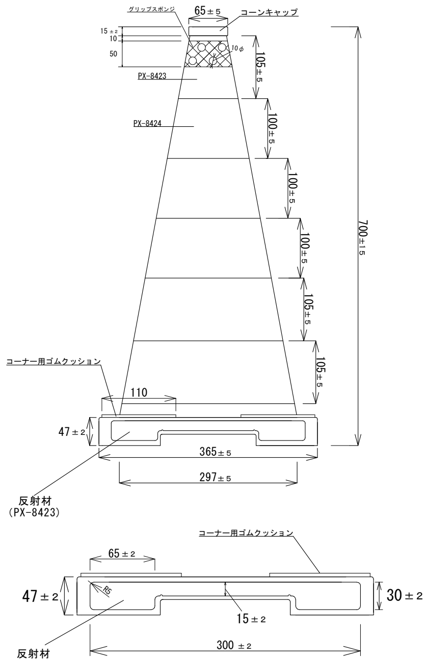
ベース部 拡大図
