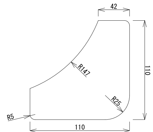
コーナー用ゴムクッション 拡大図
